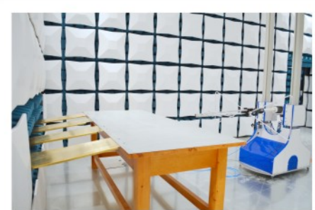
■ 汽车电子产品测试桌
